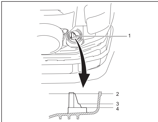
► 1. Medidor de nivel de aceite 2. Marca de límite superior 3. Nivel de 100 ml (3,4 onzas líquidas) 4. Marca de límite inferior
