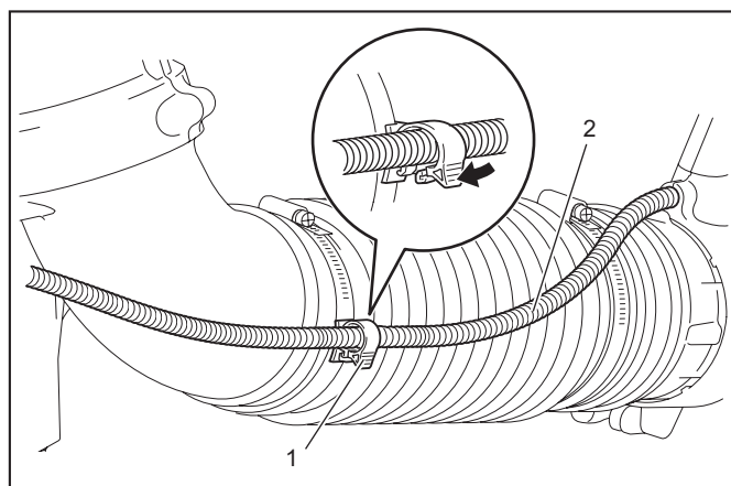
► 1. Porte-câble 2. Câble de contrôle
