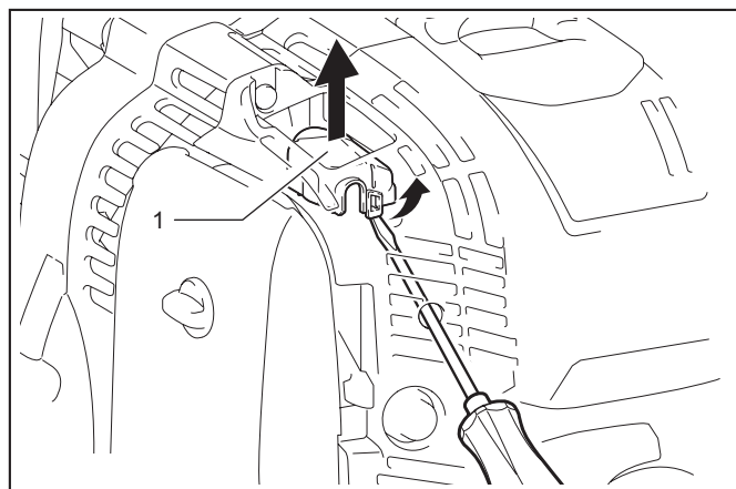
► 1. Couvercle de carburateur
