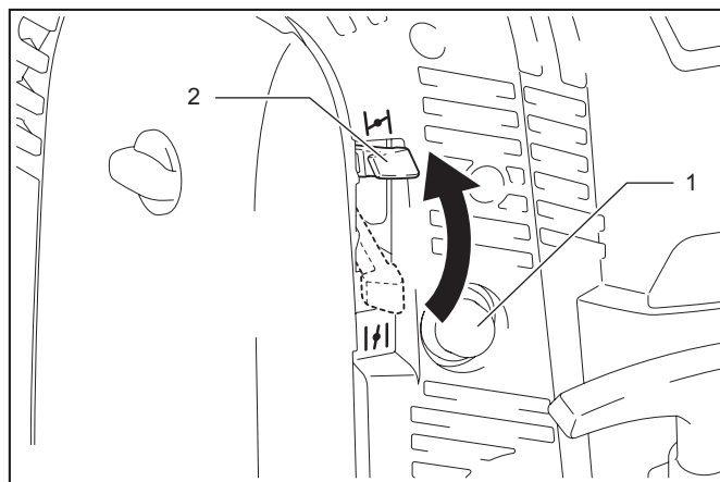
► 1. Bomba cebadora 2. Palanca del ahogador
