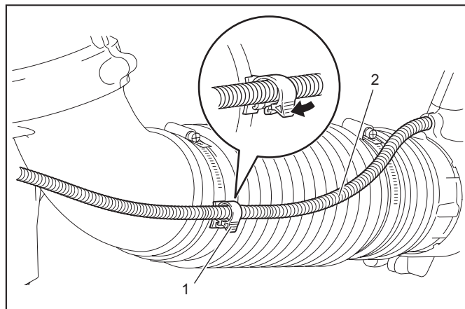
► 1. Sujetacables 2. Cable de control
