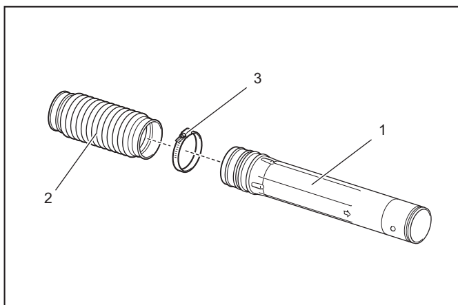
► 1. Tubo de la rótula 2. Tubo flexible 3. Abrazadera para manguera
