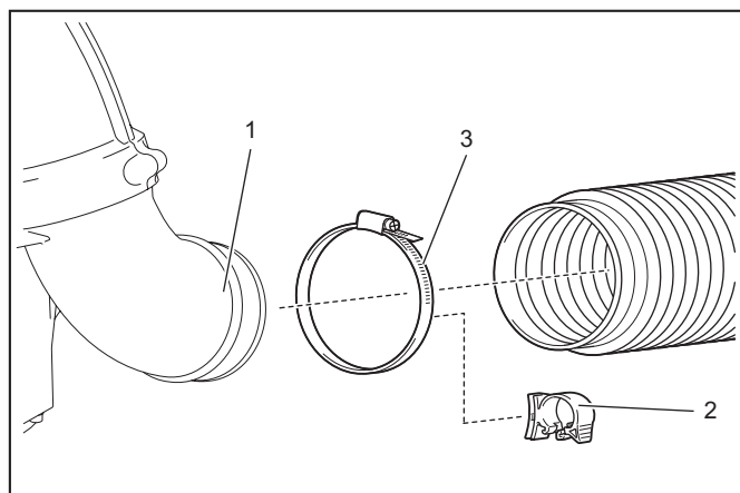
► 1. Codo 2. Sujetacables 3. Abrazadera para manguera
