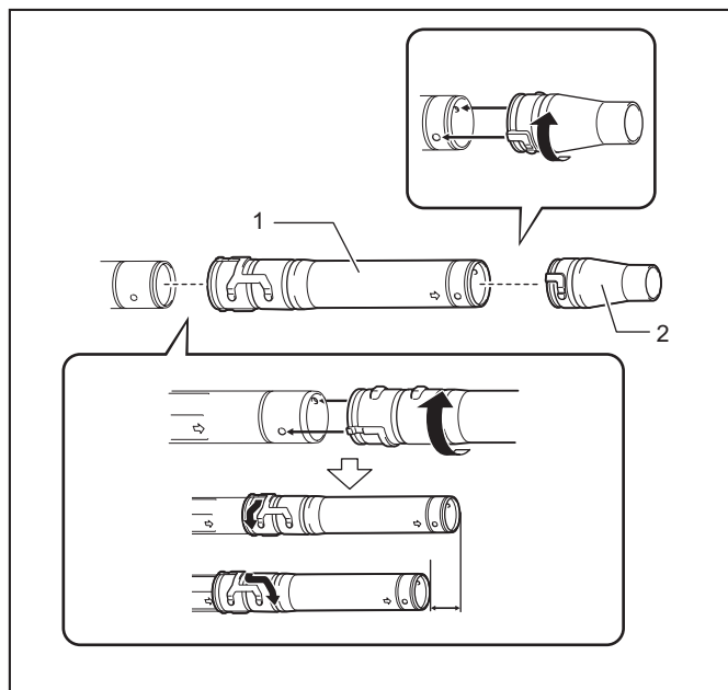
► 1. Tubo largo/corto 2. Boquilla de la sopladora
